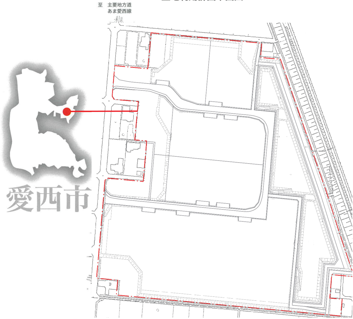
土地利用計画平面図
