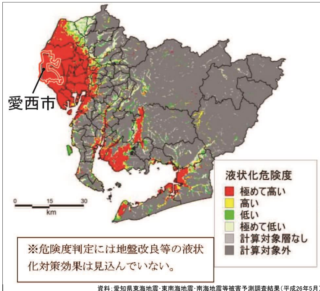
図：理論上最大想定モデルの地震(陸側ケース)の液状化危険度予測結果
