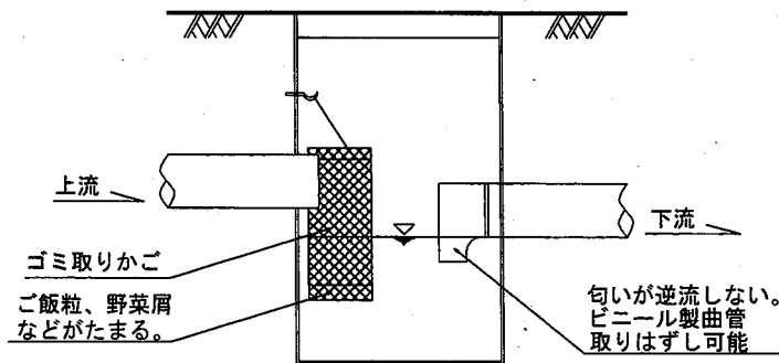
分離ます（φ300）構造図（例）
