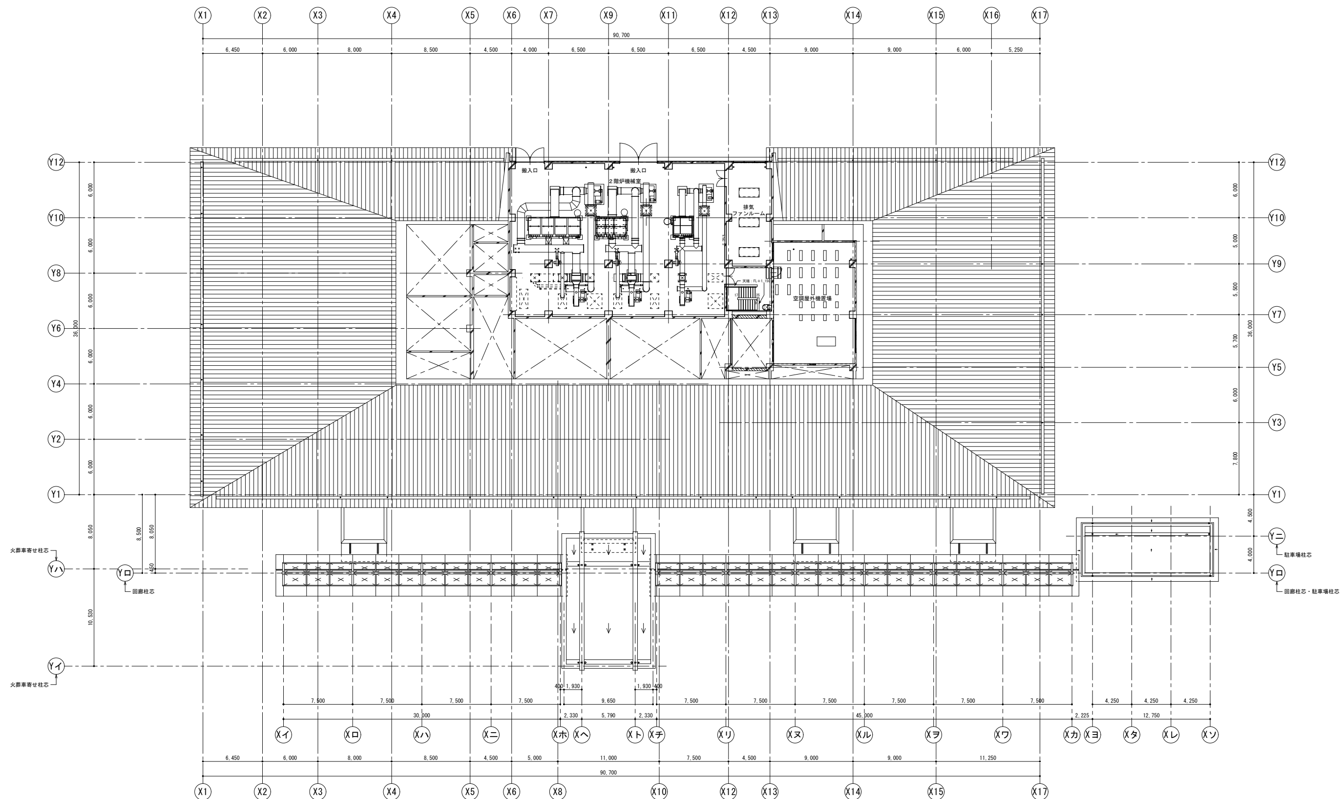
2階 平面図
