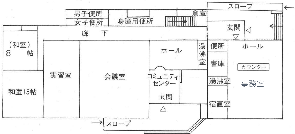
1 階 平 面 図
