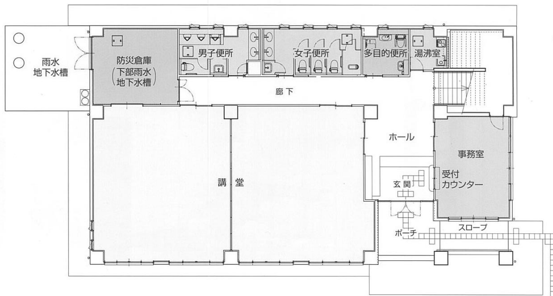
1階平面図
