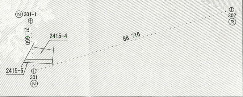
引照点配点図 (1/1000)
